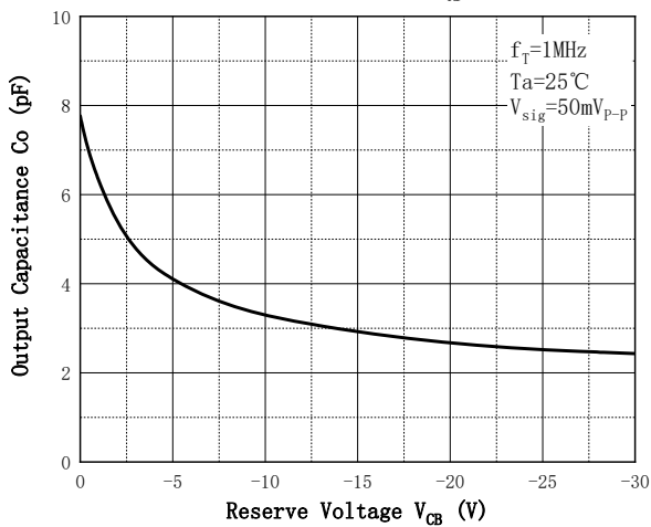
Fig.5 - C o — V CB
